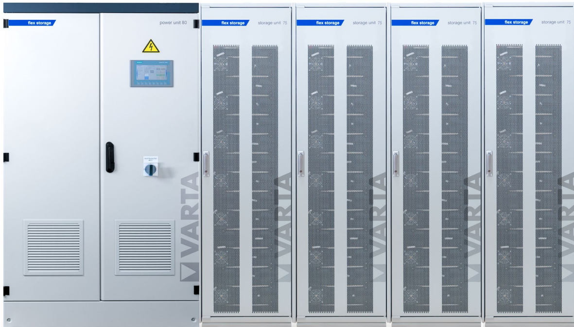
Abbildung 1: E 80/300 (115A ES) –beispielhafte Darstellung (Abbildung ähnlich)
