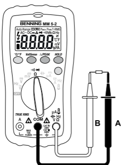
Bild 6: Widerstandsmessung Fig. 6: Resistance measurement Fig. 6: Mesure de résistance Fig. 6: Medición de resistencia Obr. 6: Μέτρηση odporu σχήμα 6: Μέτρηση αντίστασης ill. 6: Misura di resistenza Fig. 6: Weerstandsmeting Rys.6: Pomiar rezystancji Рис. 6: Измерение сопротивления Resim 6: Direnç Ölçümü
