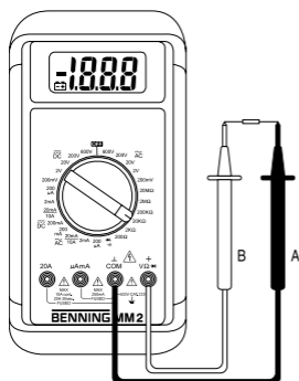
Bild 6: Widerstandsmessung Fig. 6: Resistance measurement Fig. 6: Mesure de résistance Fig. 6: Medición de resistencia Obr.6: Měření odporu σχήμα 6: Μέτρηση αντίστασης ill. 6: Misura di resistenza Fig. 6: Weerstandsmeting Rys.6: Pomiar rezystancji Imaginea 6: Măsurarea rezistenței Рис. 6: Измерение сопротивления Fig. 6: Resistansmätning Resim 6: Direnç Ölçümü
