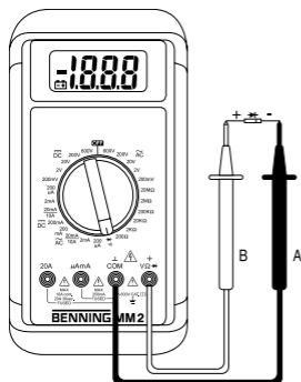
Bild 7: Diodenprüfung Fig. 7: Diode Testing Fig. 7: Contrôle de diodes Fig. 7: Verificación de diodos Obr. 7: Měření diod σχήμα 7: Έλεγχος διόδου ill. 7: Prova diodi Fig. 7: Diodecontrole Rys.7: Pomiar diody Imaginea 7: Măsurarea diodelor Рис. 7: Проверка диодов Fig. 7: Diod-test Resim 7: Diyot kontrolü
