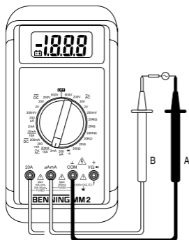
Bild 5: Wechselstrommessung Fig. 5: AC current measurement Fig. 5: Mesure de courant alternatif Fig. 5: Medición de corriente alterna Obr.5: Měření střídavého proudu σχήμα 5: μέτρηση εναλλασσόμενου ρεύματος ill. 5: Misura corrente alternata Fig. 5: Meten van wisselstroom Rys.5: Pomiar prądu przemiennego Imaginea 5: Măsurarea curentului alternativ Рис. 5: Измерение переменного тока Fig. 5: Genomgångstest med summer Resim 5: Alternatif Akım Ölçümü
