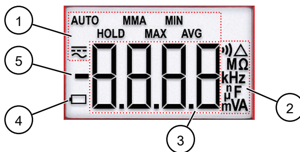
Abb. 8: Digitalanzeige
