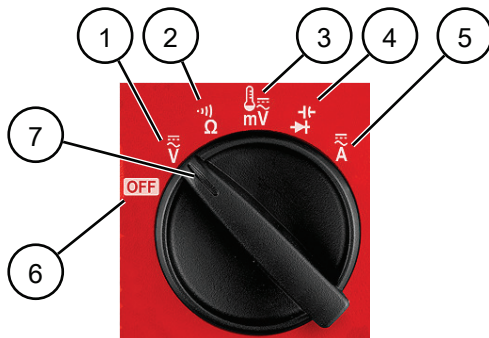
Abb. 7: Drehschalter
