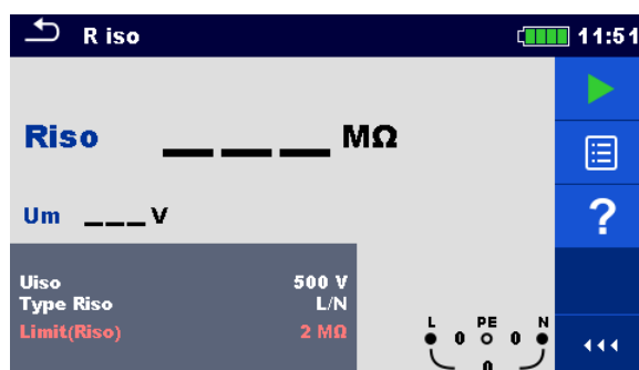
Abbildung 4.6: Menü Isolationswiderstandsmessung
