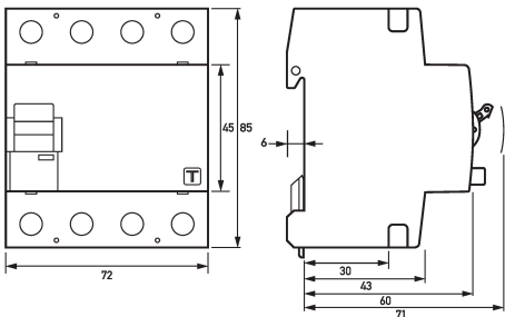
Maßzeichnung Fehlerstromschutzschalter DFS 4 016-4/0,03-B SK MI HD
