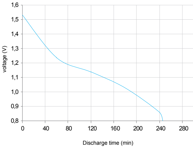
Toy 1h/d 5,1 ohm cutoff 0,8 V
