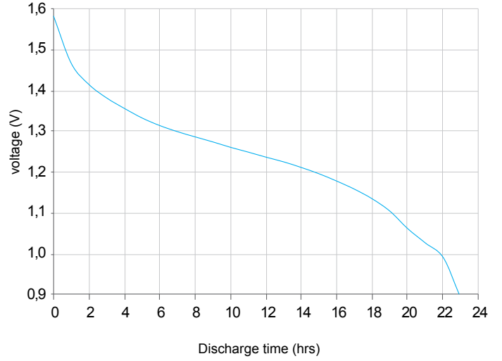
Digital audio 1h/12h 50 mA cutoff 0,9 V
