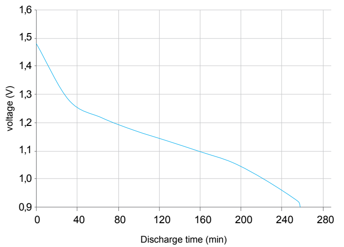
Portable lighting 4m/h 8h/d 5,1 ohm cutoff 0,9 V
