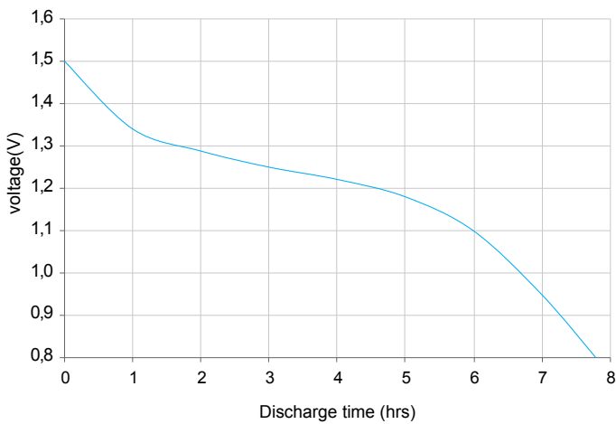
Motor/Toy 1h/d 3,9 ohm cutoff 0,8 V
