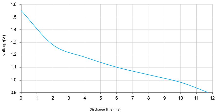
Portable stereo 2h/d 400 mA cutoff 0,9 V
