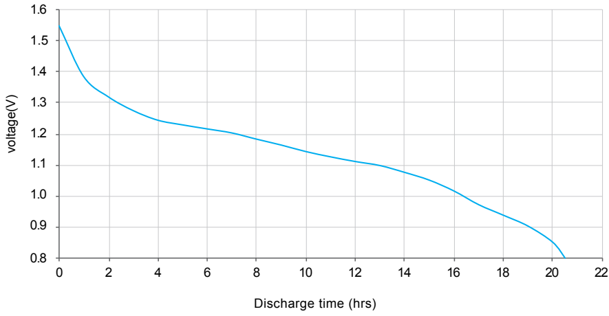
Toy 1h/d 3,9 ohm cutoff 0,8 V
