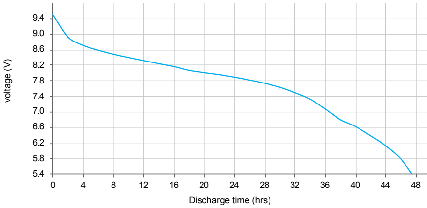
Clock radio 2h/d 620 ohm cutoff 5,4 V
