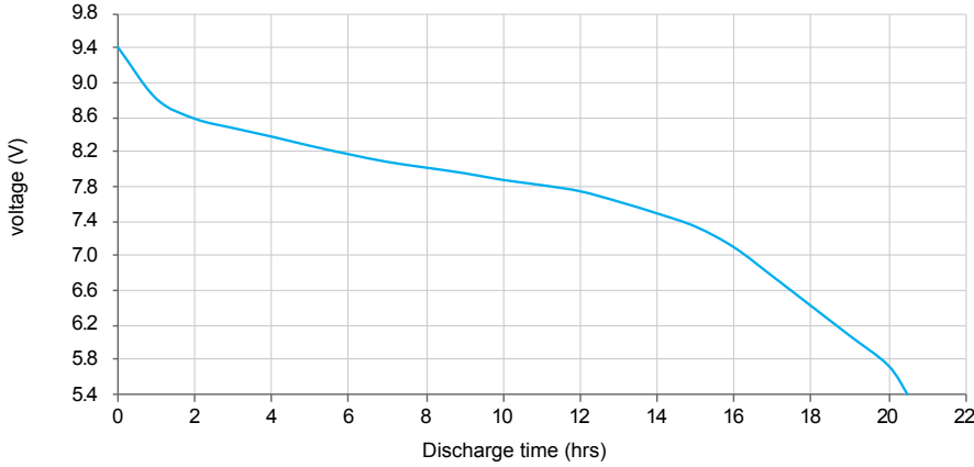
Toy 1h/d 270 ohm cutoff 5,4 V
