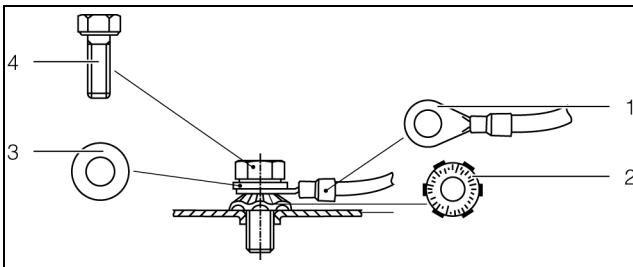
Bild 15: Potentialutjämnings utförande
