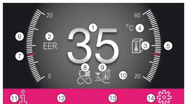
Bild 18: Startskärmens uppbyggnad
