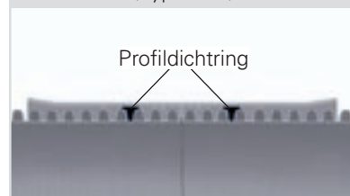
Profildichtring im dritten Wellental
