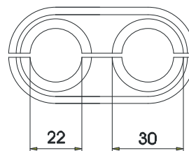
Kabelzugang
