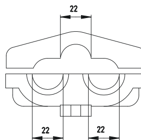
Kabelzugang
