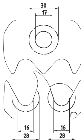
Kabelzugang
