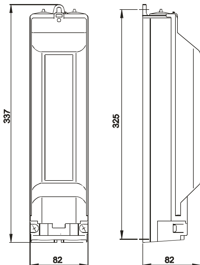
Kabelzugang
