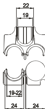
Kabelzugang
