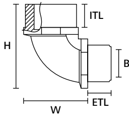
HelaGuard 90° Anschlusswinkel
