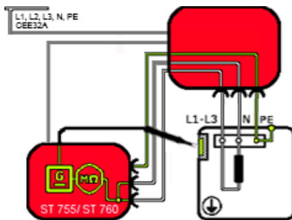
Stromlaufplan
