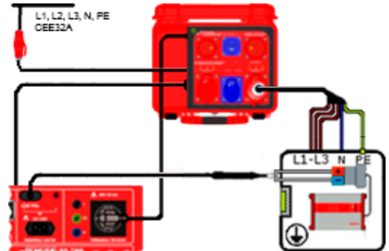
Anschlusschema
