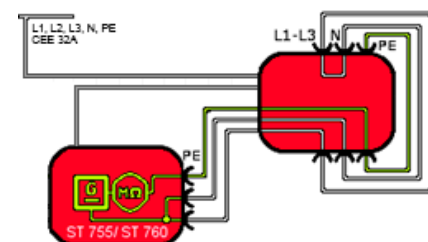
Stromlaufplan
