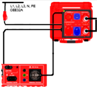
Anschlusschema
