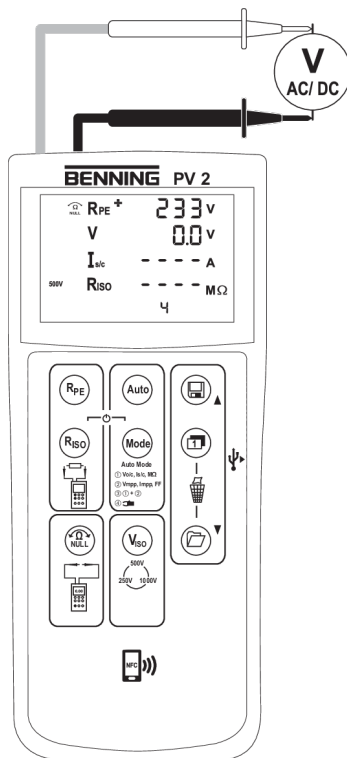
Abb. 8: Gleich- und Wechselspannungsmessung
