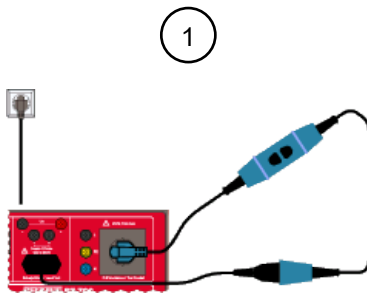
Abb. 16: PRCD prüfen (Anschlusschema)
