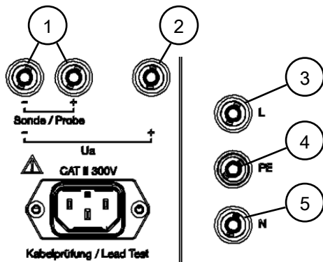
Abb. 5: Geräteansicht-Buchsen
