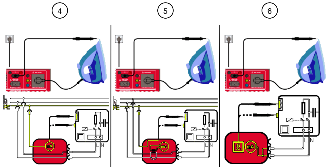
Abb. 12: Berührungsstrom prüfen SK II (Anschlussschema beispielhaft für VDE 0701 und VDE 0702, Stromlaufplan)
