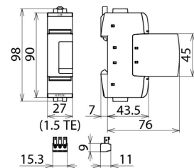
Maßbild DG SE CI WE 440 FM
