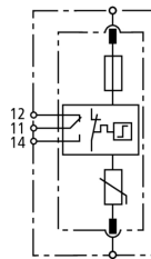
Principalschaltbild DG SE CI WE 440 FM
