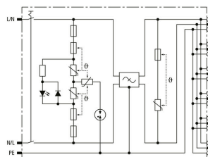
Principalschaltbild SFL PRO 6X
