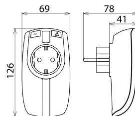
Maßbild DPRO 230
