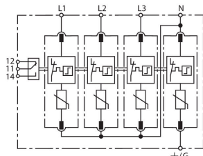
Prinzipschaltbild DG MU 3PY 480 4W+G R
