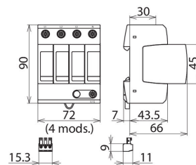
Maßbild DG MU 3PY 480 4W+G R
