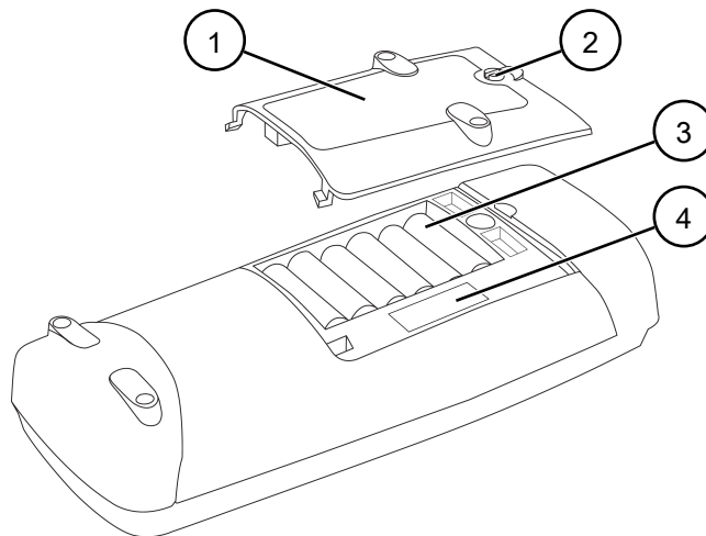
Abb. 13: Batteriewechsel (beispielhaft)
