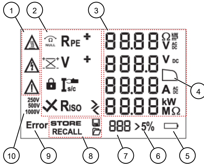
Abb. 2: Digitalanzeige
