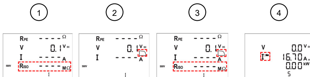
Abb. 3: Modi
