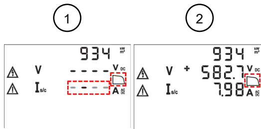
Abb. 4: Kennlinienmessung im Mode 2 und 3
