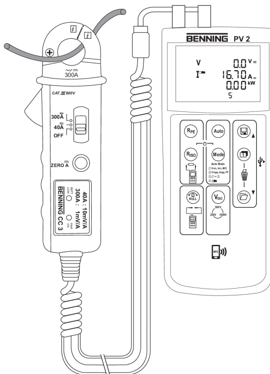
Abb. 9: Strommessung mit optionalem BENNING CC 3
