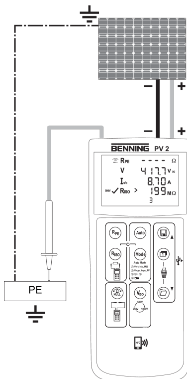
Abb. 7: Automatische PV-Messung
