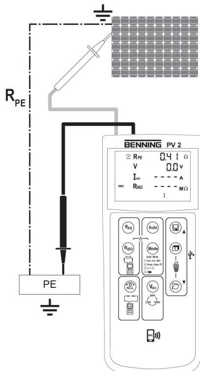
Abb. 6: Schutzleiterwiderstand messen
