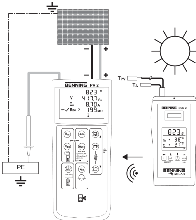
Abb. 12: Funkverbindung zum BENNING SUN 2
