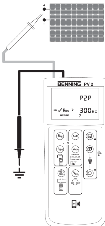
Abb. 10: Isolationswiderstand messen
