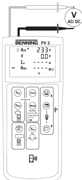
Abb. 8: Gleich- und Wechselspannungsmessung
