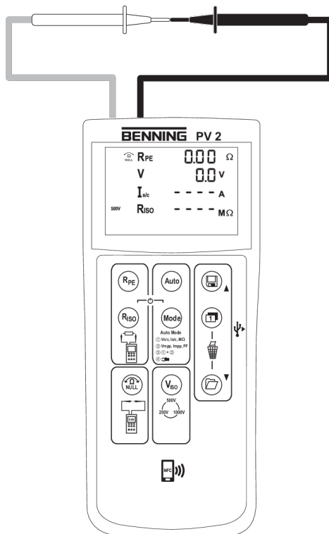
Abb. 5: Nullabgleich der 4 mm-Sicherheitsmessleitungen
