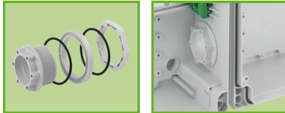
Abbildung 14: Kombiverschraubung
