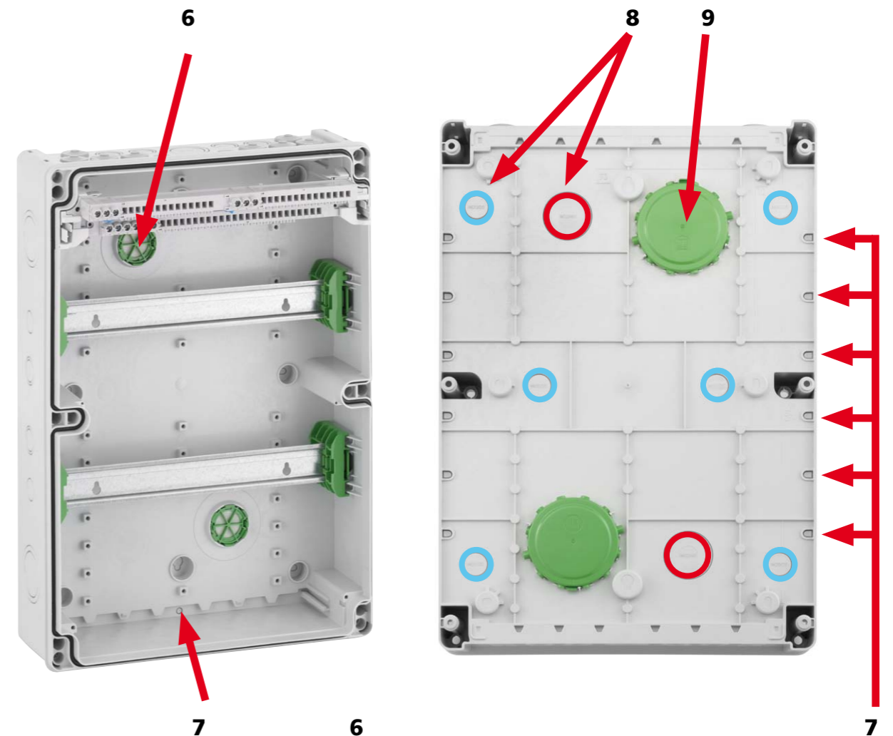
Abbildung 3: Kastenboden Vorderseite, Rückseite (Bild 2)
