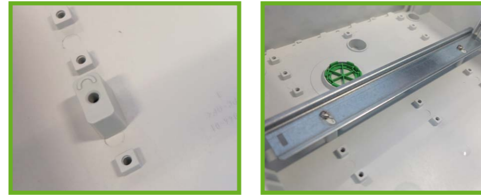
Abbildung 31: Universelle Bodenbefestigung
