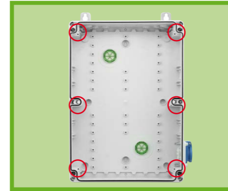
Abbildung 25: Befestigungspunkte außerhalb des Dichtbereichs
