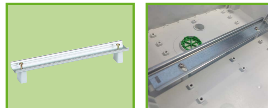
Abbildung 18: Normschiene mit universeller Bodenbefestigung
