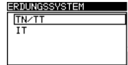
Abbildung 4.8: Auswahl des Erdungssystems
