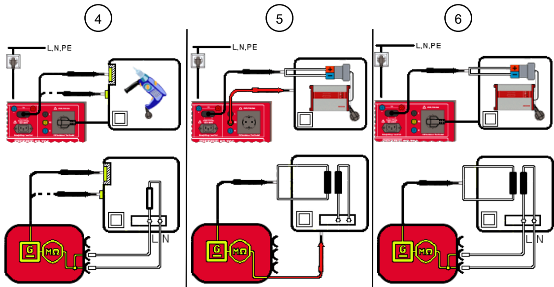
Illustration 15: Contrôler la résistance d'isolement, Classe II (schéma de raccordement exemplaire pour EN 50678 et EN 50699, schéma électrique)
