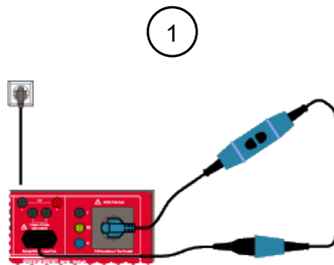
Illustration 28: Contrôler les PRCD (schéma de raccordement)
