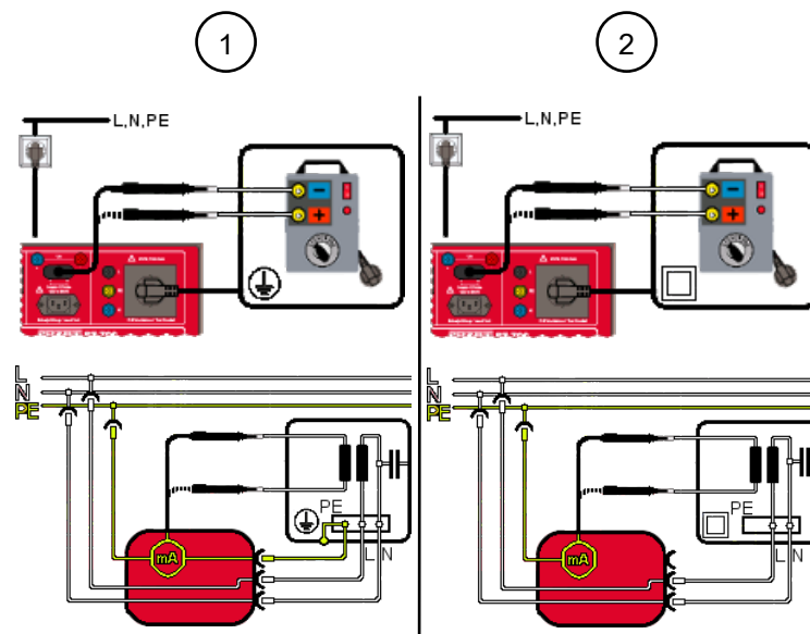
Illustration 27: Contrôler le courant de contact du circuit de soudage (schéma de raccordement, schéma électrique)
