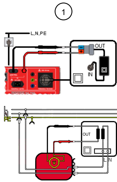
Illustration 25: Contrôler la très basse tension de protection, Classe I (schéma de raccordement, schéma électrique)
