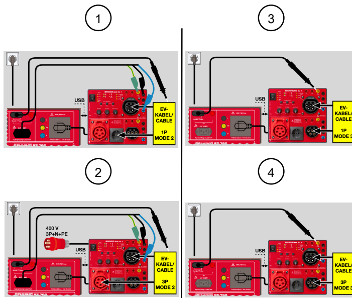
Illustration 29: Contrôle EVSE (schéma de raccordement du montage d'essai EVSE)
