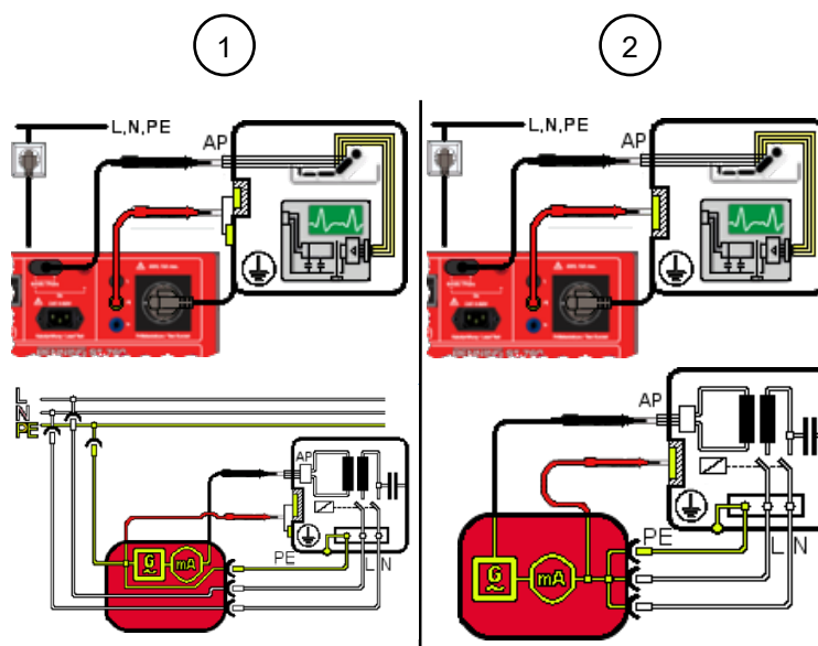
Illustration 21: Contrôler le courant de fuite patient, Classe I (schéma de raccordement pour EN 62353, schéma électrique, partie appliquée type F)
