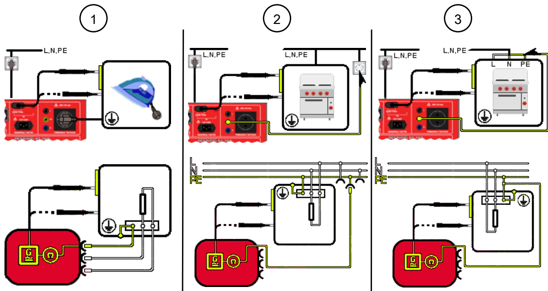
Illustration 13: Contrôler la résistance du conducteur de protection (schéma de raccordement exemplaire pour EN 50678 et EN 50699, schéma électrique)
