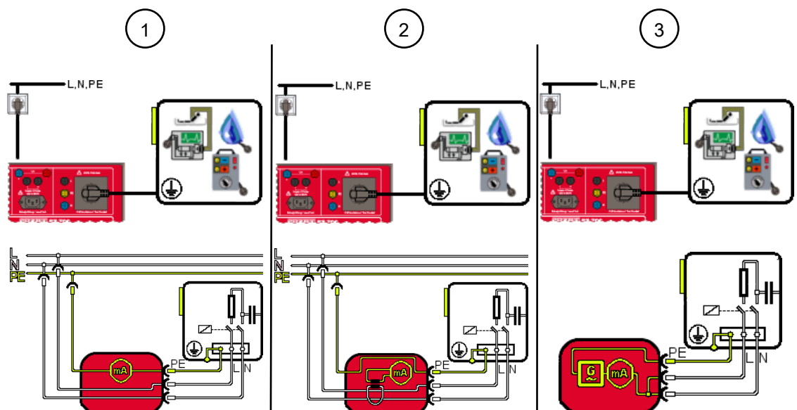
Illustration 17: Contrôler le courant du conducteur de protection (schéma de raccordement, schéma électrique)
