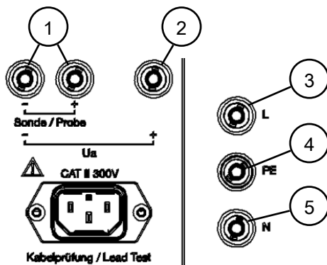
Illustration 12: Vue de l'appareil – Douilles
