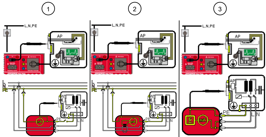
Illustration 20: Contrôler le courant de fuite appareil (schéma de raccordement pour EN 62353, schéma électrique)
