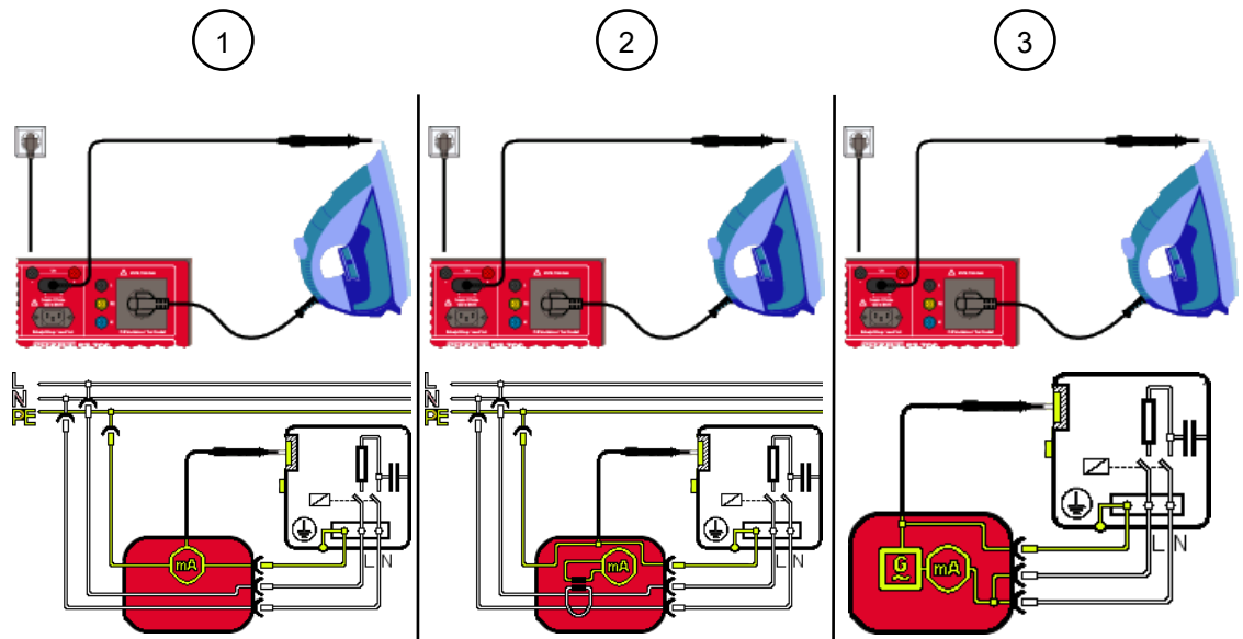
Illustration 18: Contrôler le courant de contact, Classe I (schéma de raccordement exemplaire pour EN 50678 et EN 50699, schéma électrique)
