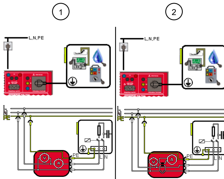
Illustration 23: Contrôle de fonctionnement (schéma de raccordement, schéma électrique)
