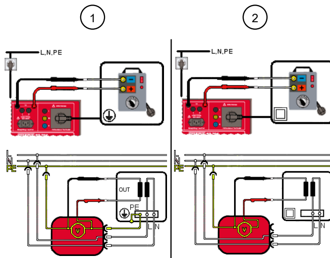
Illustration 26: Contrôler la tension du circuit de soudage (schéma de raccordement, schéma électrique)
