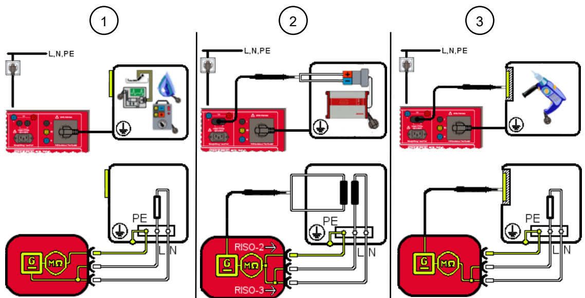
Illustration 14: Contrôler la résistance d'isolement, Classe I (schéma de raccordement exemplaire pour EN 50678 et EN 50699, schéma électrique)
