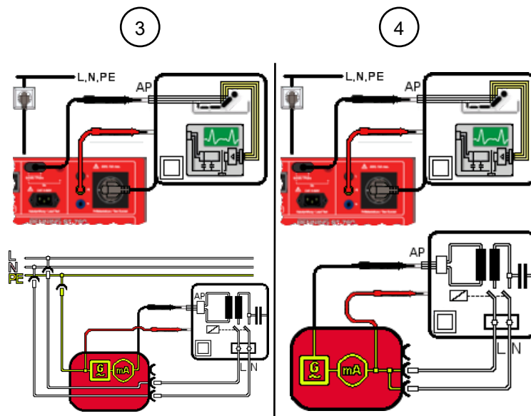
Illustration 22: Contrôler le courant de fuite patient, Classe II (schéma de raccordement pour EN 62353, schéma électrique, partie appliquée type F)
