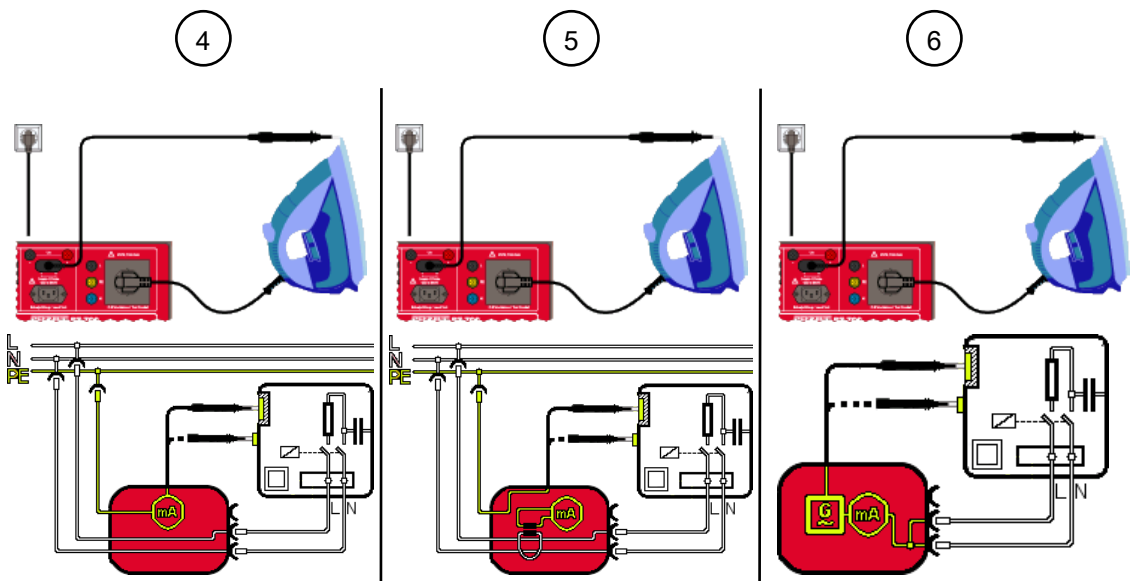
Illustration 19: Contrôler le courant de contact, Classe II (schéma de raccordement exemplaire pour EN 50678 et EN 50699, schéma électrique)
