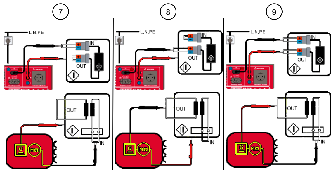
Illustration 16: Contrôler la résistance d'isolement, Classe III (schéma de raccordement exemplaire pour EN 50678 et EN 50699, schéma électrique)
