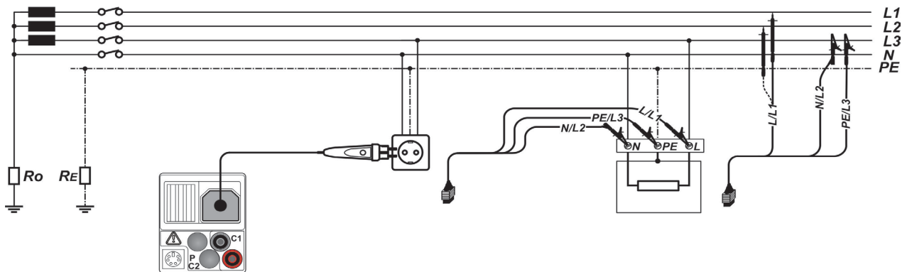
Afbeelding 5.28: Aansluiting van de optionele Commander-teststekker (044149) en van de 3-geleider testdraad - Afbeelding met IT 130 als voorbeeld
