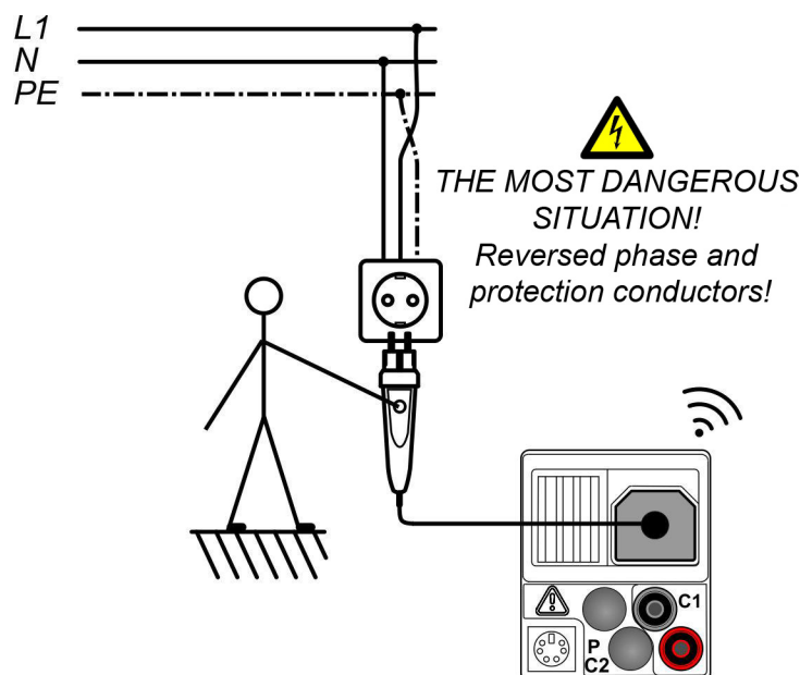
Afbeelding C.4: Verwisselde L- en PE-geleider – fasespanning op PE-aansluiting wordt herkend door de TEST-toets op de optionele Commander-teststekker (044149) aan te raken. - Afbeelding met IT 130 als voorbeeld
