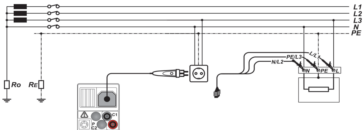
Afbeelding 5.24: Aansluiting van de optionele Commander-teststekker (044149) en van de 3-geleider testdraad - Afbeelding met IT 130 als voorbeeld
