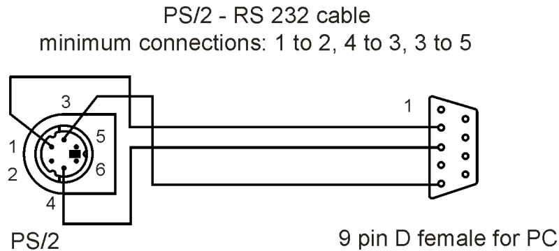
Afbeelding 6.14: PIN-aansluiting van de seriële RS 232-kabel - Afbeelding met IT 130 als voorbeeld
