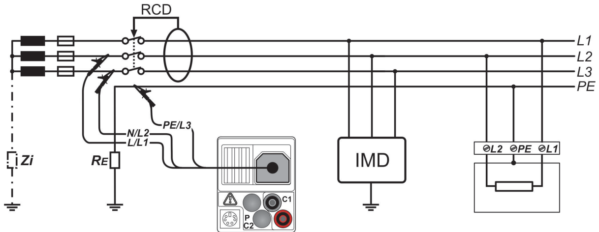
Afbeelding 5.43: Aansluiting van de 3-geleider testdraad in RCD-beveiligde installatie - Afbeelding met IT 130 als voorbeeld
