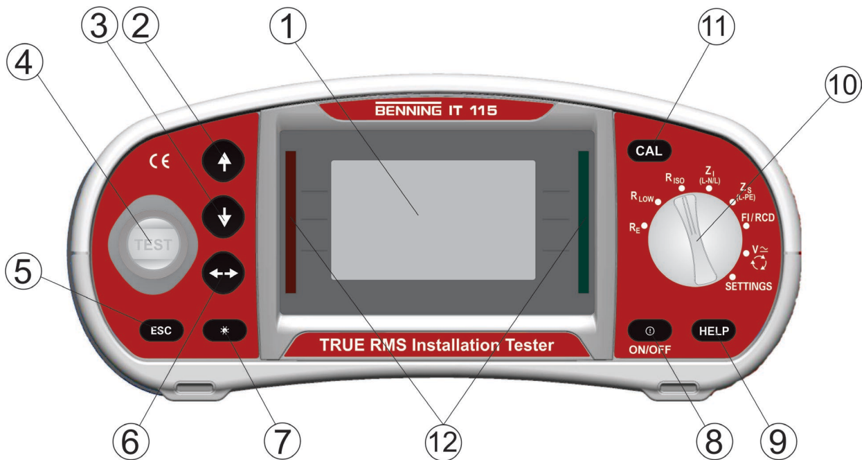
Afbeelding 3.1: Voorzijde (IT 115)
