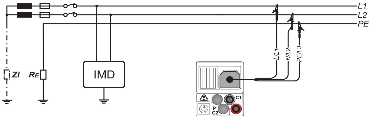
Afbeelding 5.42: Aansluiting van de 3-geleider testdraad - Afbeelding met IT 130 als voorbeeld
