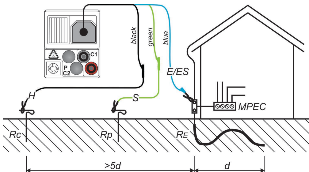
Afbeelding 5.33: Aansluiting van de optionele aardingsset (044113) - meting van de hoofdaarding - Afbeelding met IT 130 als voorbeeld
