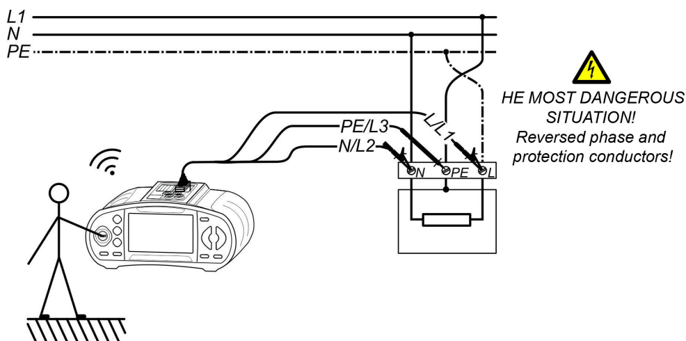
Afbeelding 5.37: Omgewisselde L- en PE-geleider – fasespanning op de PE-geleider wordt herkend door de TEST-toets op het apparaat aan te raken.
