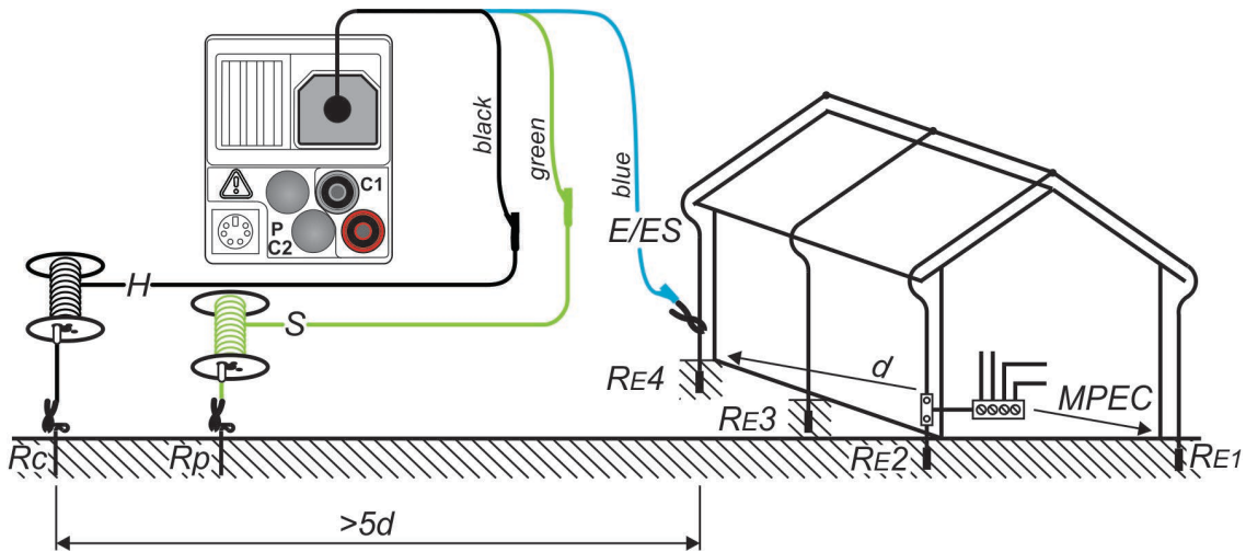
Afbeelding 5.34: Aansluiting van de optionele aardingsset (044113) - meting aan de bliksemafleider - Afbeelding met IT 130 als voorbeeld
