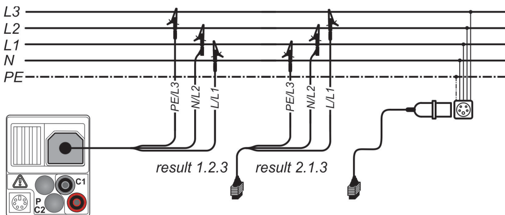
Afbeelding 5.2: Aansluiting van 3-geleider testdraad en optionele CEE-meetadapter (044148) in driefasesysteem - Afbeelding met IT 130 als voorbeeld
