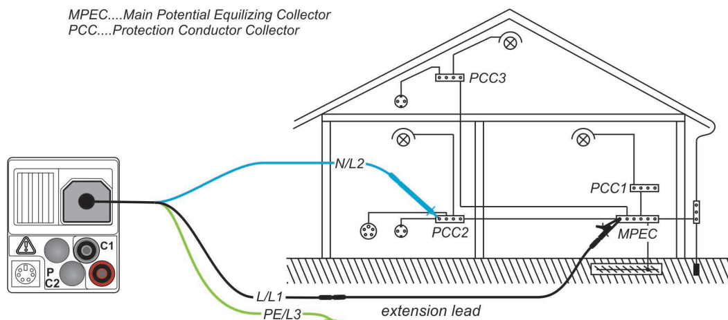
Afbeelding 5.9: Aansluiting van de 3-geleider testdraad en de optionele 40 m meetkabel BENNING TA 5 (044039) - Afbeelding met IT 130 als voorbeeld
