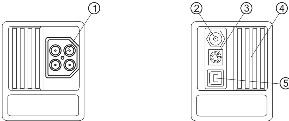
Afbeelding 3.3: Aansluitpaneel (IT 115)
