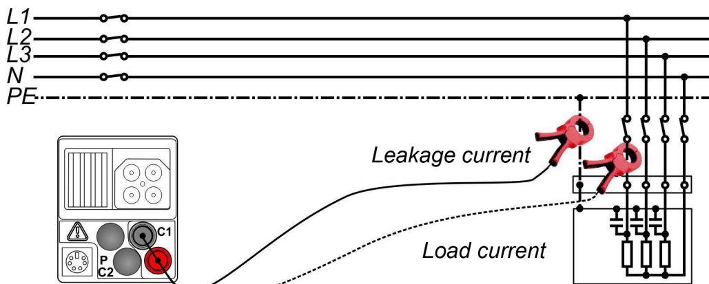
Afbeelding 5.39: Aansluiting van de optionele stroomtangadapter BENNING CC 1 of BENNING CC 3 - Afbeelding met IT 130 als voorbeeld
