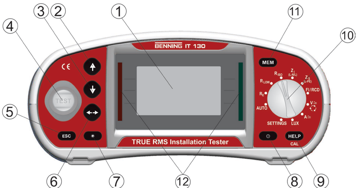
Afbeelding 3.2: Voorzijde (IT 130)
