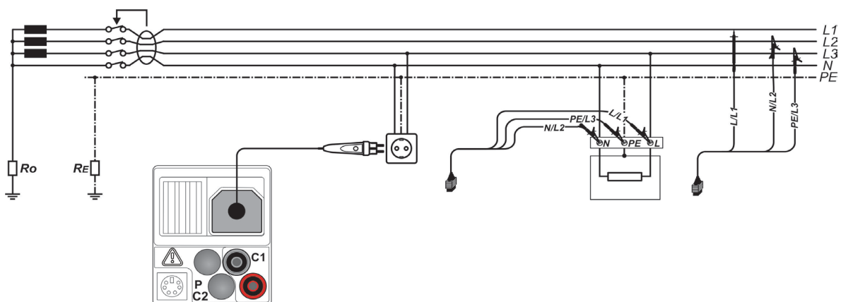
Afbeelding 5.3: Aansluiting van de optionele Commander-teststekker (044149) en de 3-geleider testdraad in het een-/driefasesysteem - Afbeelding met IT 130 als voorbeeld
