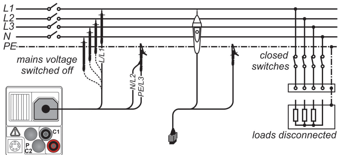
Afbeelding 5.6: Aansluiting van 3-geleider testdraad en Commander-testpen (044115) - Afbeelding met IT 130 als voorbeeld
