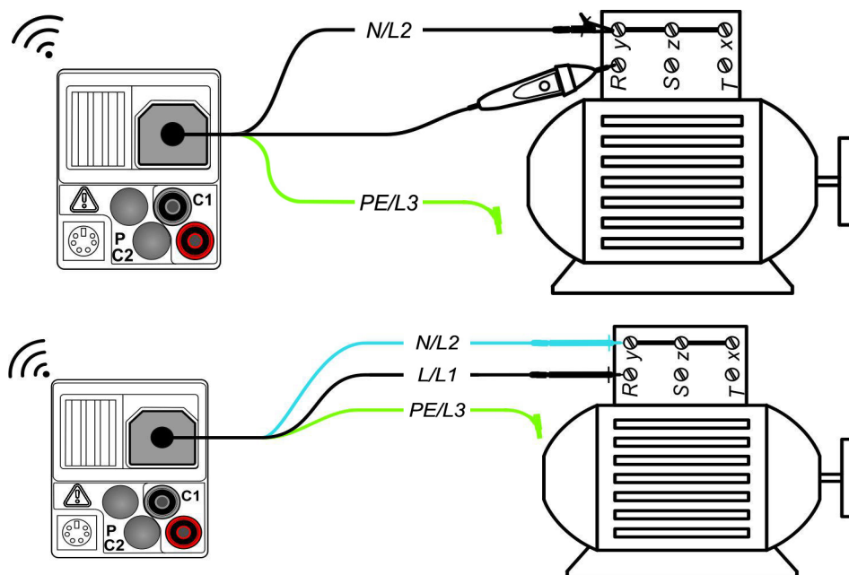
Afbeelding 5.11: Gebruik van de Commander-testpen en 3-geleider testdraad - Afbeelding met IT 130 als voorbeeld
