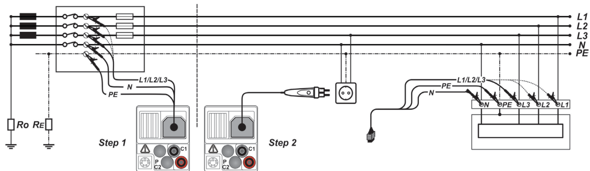
Afbeelding 5.30: Aansluiting van de optionele Commander-teststekker (044149) en van de 3-geleider testdraad - Afbeelding met IT 130 als voorbeeld
