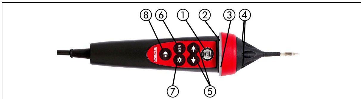
Afbeelding C.1: Voorzijde van de Commander-testpen schakelbaar met TEST-toets (044155)
