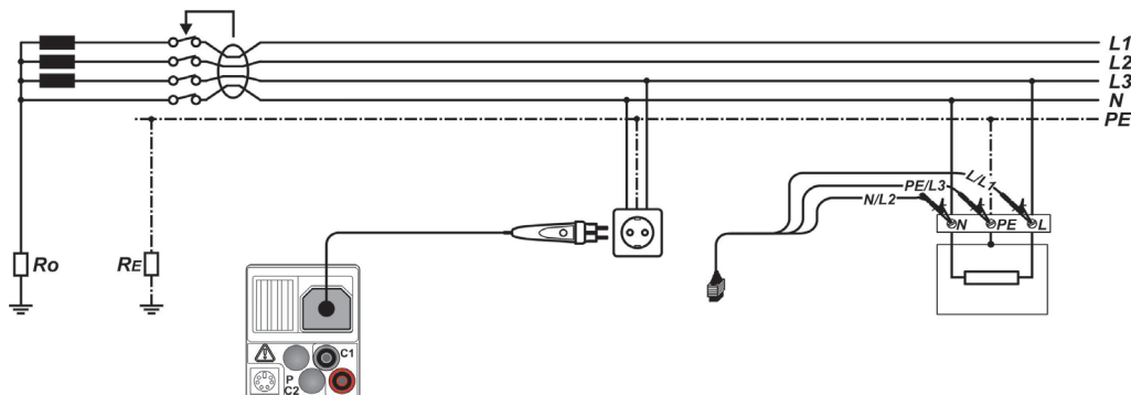
Afbeelding 5.17: Aansluiting van de optionele Commander-teststekker (044149) en van de 3-geleider testdraad - Afbeelding met IT 130 als voorbeeld
