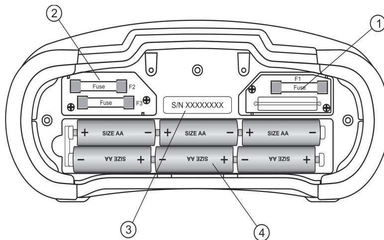
Afbeelding 3.6: Batterij- en zekeringvak
