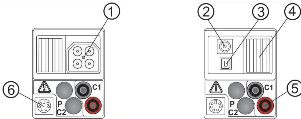
Afbeelding 3.4: Aansluitpaneel (IT 130)
