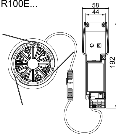
ALBA R100E...
