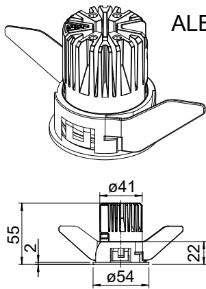
ALBA R68E...
