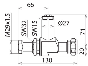
Maßbild DGA LG 7 16 MFA
