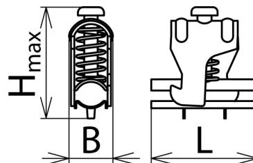
Maßbild SAK
