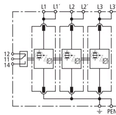
Prinzip Schaltbild DV M TNC 255 FM
