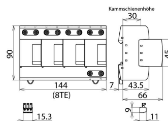
Maßbild DV M TT 255 FM
