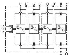
Prinzipialschaltbild DV M TT 255 FM
