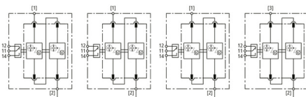
Prinzipialschaltbild DV M2 880 FM
