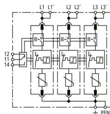
Prinzip Schaltbild DG MP TNC ACI 275 FM
