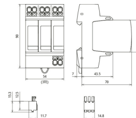
Maßbild DG MP TNC ACI 275 FM
