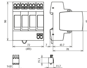
Maßbild DG MP TT ACI 385 FM
