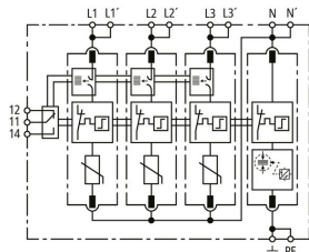
Prinzipialschaltbild DG MP TT ACI 385 FM
