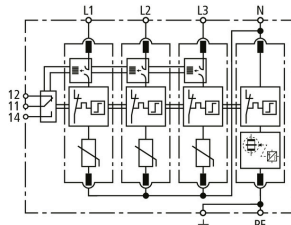
Prinzipschaltbild DG M TT ACI 275 FM
