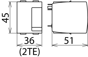
Maßbild DR MOD 4P 255 SN1871
