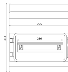
Maßbild IGA 12 IP54
