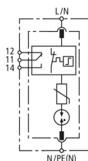
Principalschaltbild DG SE H 1000 VA FM
