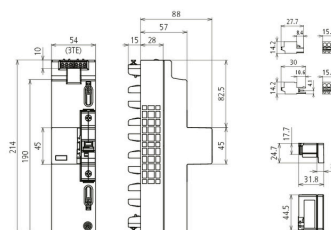
Maßbild DSH ZP 2 LSG A TT 255
