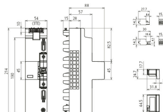
Maßbild DSH ZP B2 LSG A TT 255
