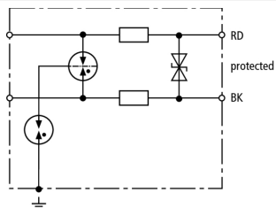
Principalschaltbild DPI MD EX 24 N 2
