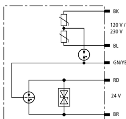
Prinzipialschaltbild DPI CD EXD 230 24 N
