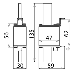
Maßbild VA NH1 280
