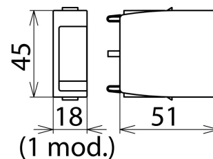
Maßbild DG PLU 230
