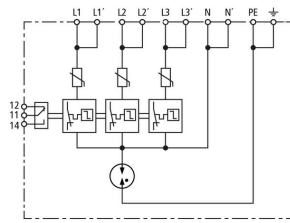
Principalschaltbild DCU EMOB 2 25
