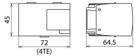
Maßbild DSE MOD NG 2P 60
