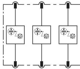
Prinzipschaltbild DSE MOD NG 2P 60
