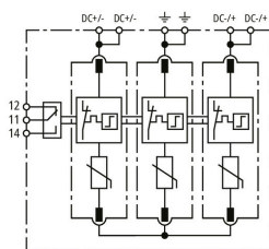
Prinzip Schaltbild DCU 2 YPV 1100 1M 1S MC4 FM
